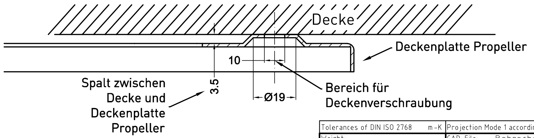
Schnitt A-A M:1:1
